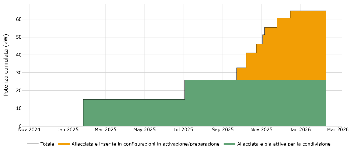
Andamento della capacità cumulata di CER Sinergie nel corso del 2025
